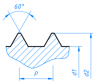
Profil navoja vijaka za pločevino
