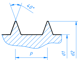
Profil navoja vijaka za iverne plošče
